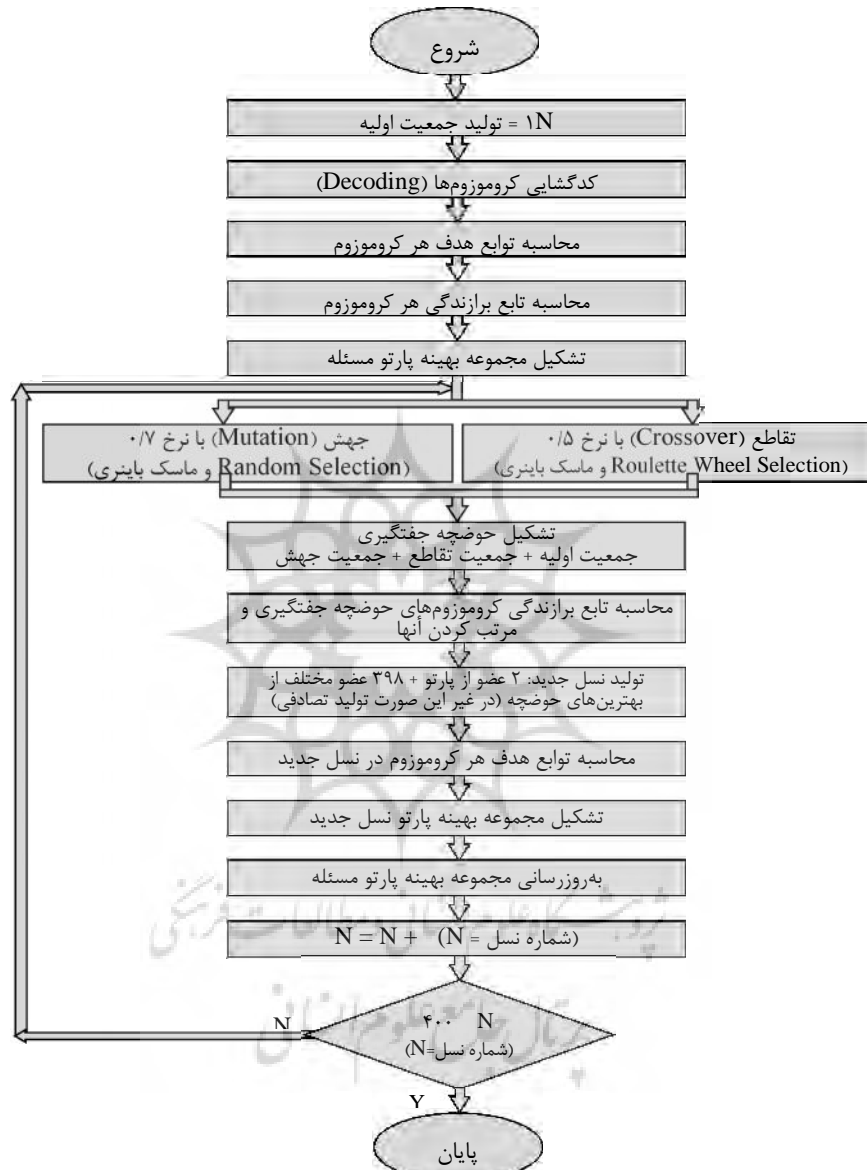
شکل ۳ فلوچارت الگوریتم MOGA
