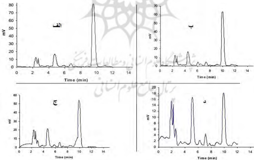
نمودار ۲: کروماتوگرام فرد ۳۰ ساله الف) پنج ساعت، ب) ۱۲ ساعت، ج) ۲۴ ساعت، د) ۳۶ ساعت بعد از مصرف تریاک (سرعت جریان یک میلی لیتر بر دقیقه، فاز متحرک ۶۵:۳۵ آب-استونیتریل، ستون نواک ۱ C 18 )
