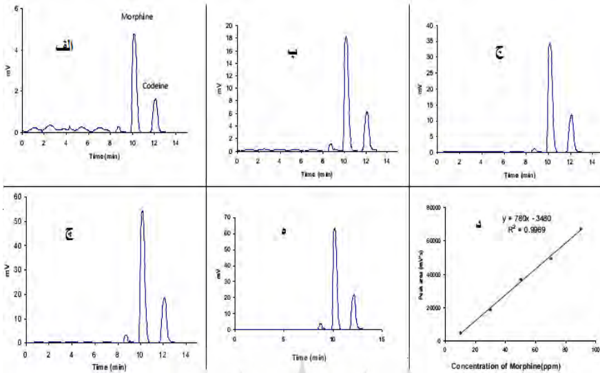
نمودار ۱: الف) کروماتوگرام محلول استاندارد ۱۰ ppm مرفین ب) ۳۰ مرفین، ج) ۵۰ ppm مرفین، چ) ۷۰ ppm مرفین، د) ۹۰ ppm مرفین، و) منحنی کالیبراسیون (سرعت جریان یک میلی لیتر بر دقیقه، فاز متحرک ۶۵:۳۵ آب-استونیتریل، ستون نواک ۱ C 18 )
