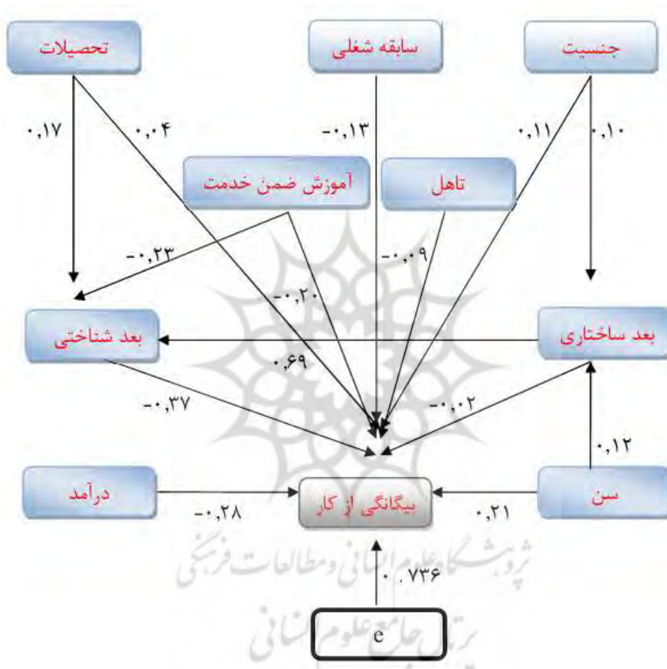
شکل ۲- مدل تحلیل مسیر متغیرهای پژوهش
