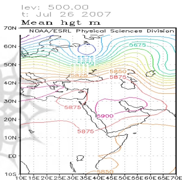
شکل ۱۲- نقشه سطح ۵۰۰ هکتوپاسکال ۱۳۸۶/۵/۴ (۲۶ جولای ۲۰۰۷) ماخذ: سایت ناسا (NCEP/NCAR)
