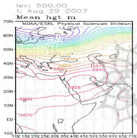
شکل ۱۳- نقشه سطح ۵۰۰ هکتوپاسکال ۱۳۸۶/۶/۷ (۲۹ آگوست ۲۰۰۷) ماخذ: سایت ناسا (NCEP/NCAR)
