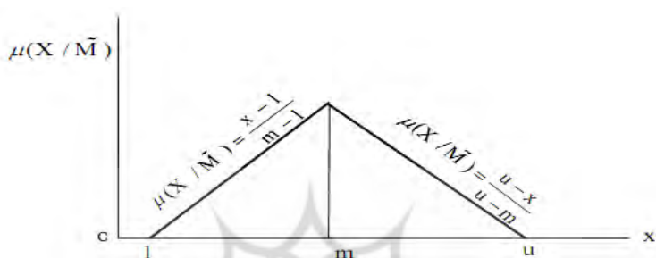
شکل 2- تابع عضویت
