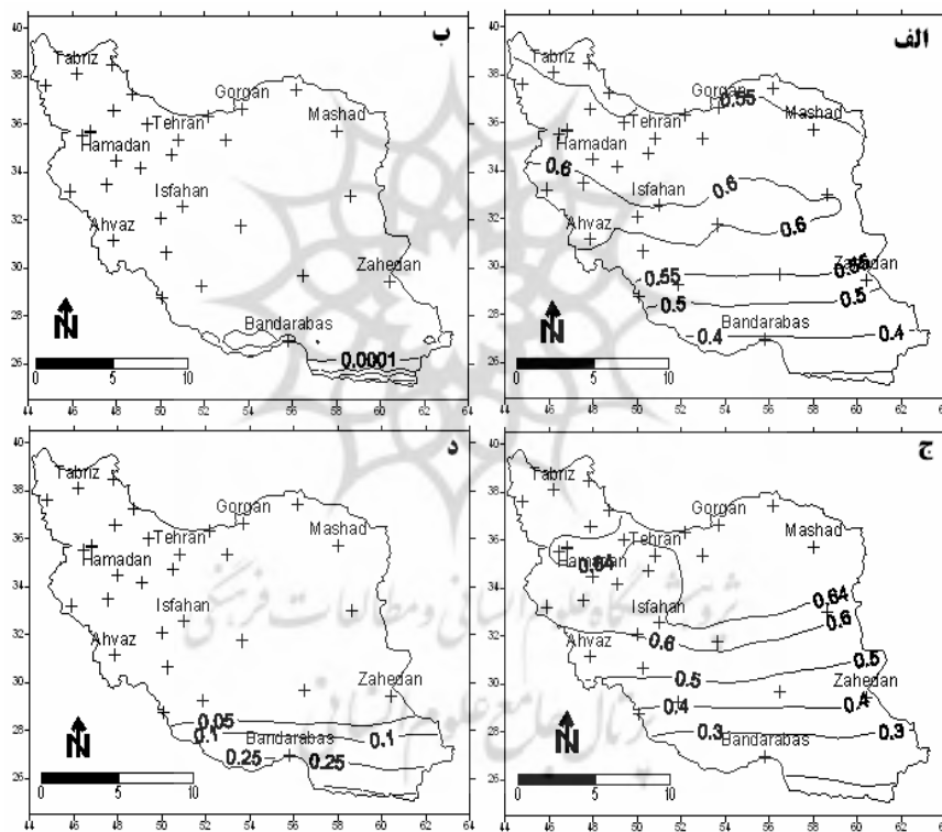
شکل (۲) توزیع ضرایب همبستگی و سطح معنی داری NINO3 با مجموع آزون در گستره ایران الف: ضرایب همبستگی همزمان ب: سطح معنی داری همزمان ج: ضرایب همبستگی با تأخیر ۱ ماهه و د: سطح معنی داری با تأخیر ۱ ماهه
