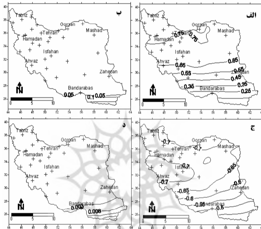
شکل (۱) توزیع ضرایب همبستگی و سطح معنی‌داری NINO1+2 با مجموع آزون در گستره ایران الف: ضرایب همبستگی ب: سطح معنی‌داری همزمان، ج: ضرایب با تأخیر ۵ ماهه و د: سطح معنی‌داری با تأخیر ۵ ماهه.
