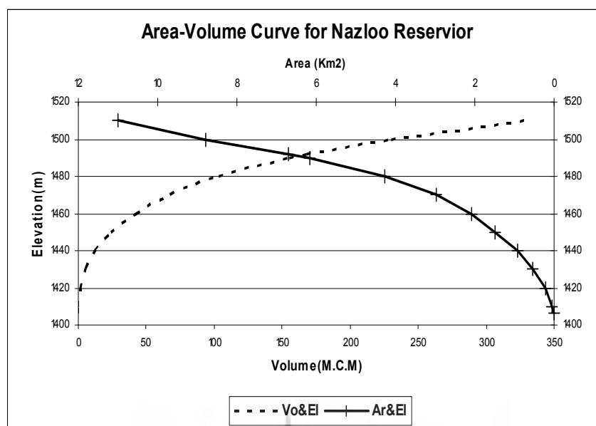
شکل ۲: منحنی سطح - حجم - ارتفاع سد نازلو در شرایط آبی
