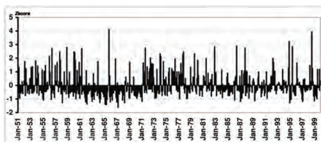
نگاره ۶: نمودار نمرات استاندارد شده بارش ماهانه حوضه
