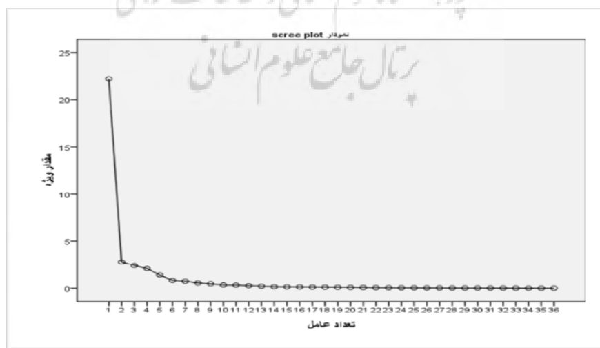
شکل ۲: نمودار Scree Plot برای تعیین تعداد عواملها
