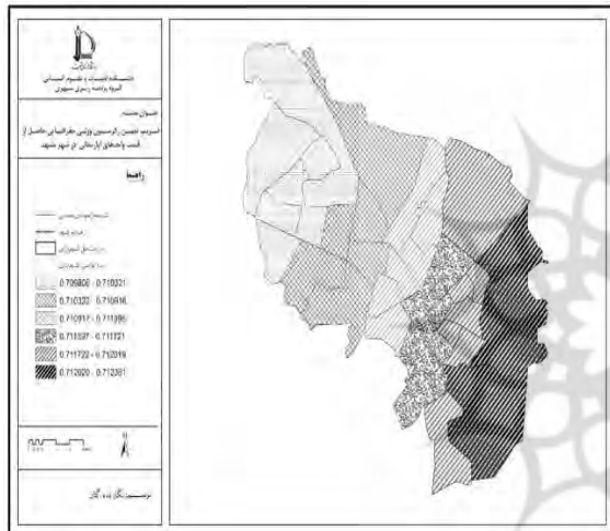
شکل ۵. Local R^2 قیمت منازل ویلایی در شهر مشهد
