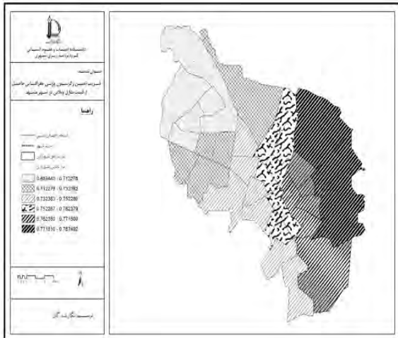
شکل ۴. Local R^2 قیمت واحدهای آپارتمانی در شهر مشهد
