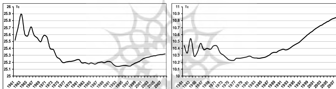
شکل ۹: میانگین شناور سری زمانی دمای کمینه ایران
