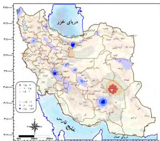
شکل ۵: شیب روند دمای بیشینه برحسب درجه در دهه مأخذ: مطالعات میدانی نگارنده، ۱۳۹۱
