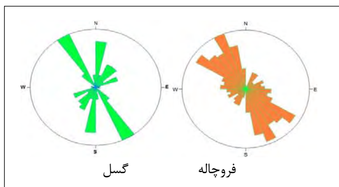
شکل ۷: نمودار گلسرخشی کشیدگی محور اصلی فروچاله‌ها و گسل‌ها
