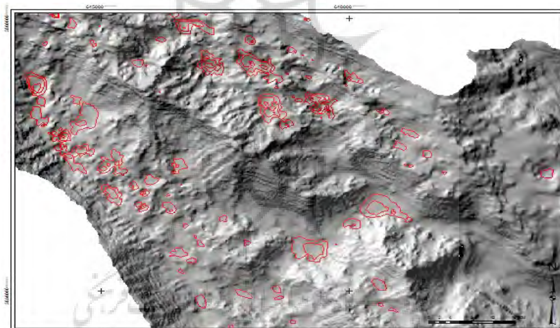
شکل ۴: انواع فروچاله‌ها در منطقه گازورخانی بر اساس مورفولوژی - برگرفته از ۱۰dem متر منطقه
