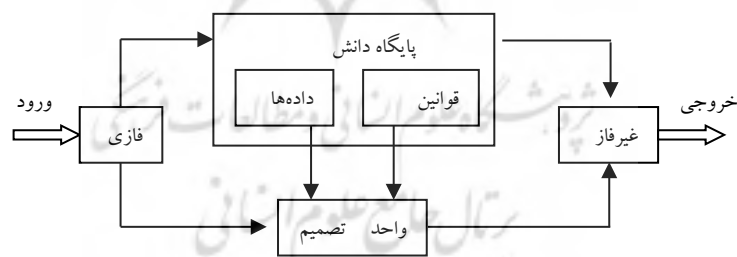
شکل ۲: ساختار کلی یک سیستم فازی
