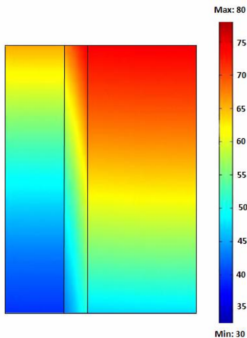
شکل ۶) توزیع دما در طول مدول، دمای جریان سیال سرد ورودی (30 °C) و دمای گاز ورودی (80 °C)
