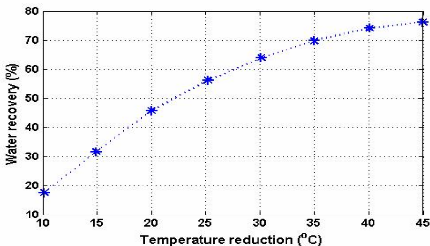
شکل ۹) نمودار درصد بازیافت آب برحسب کاهش دمای گاز دودکش (درصد آب ۱۱ ، دمای گاز دودکش 80\text{ }^{\circ}\text{C} ، دمای سیال سرد 25\text{ }^{\circ}\text{C} )
