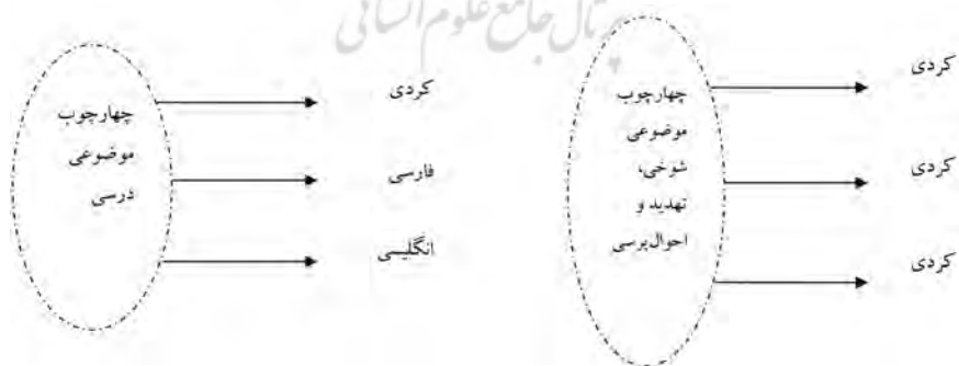
شکل ۲. رمزگردانی استعاری
