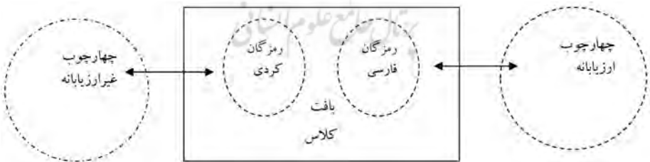
شکل ۱. رمزگردانی موقعیتی
