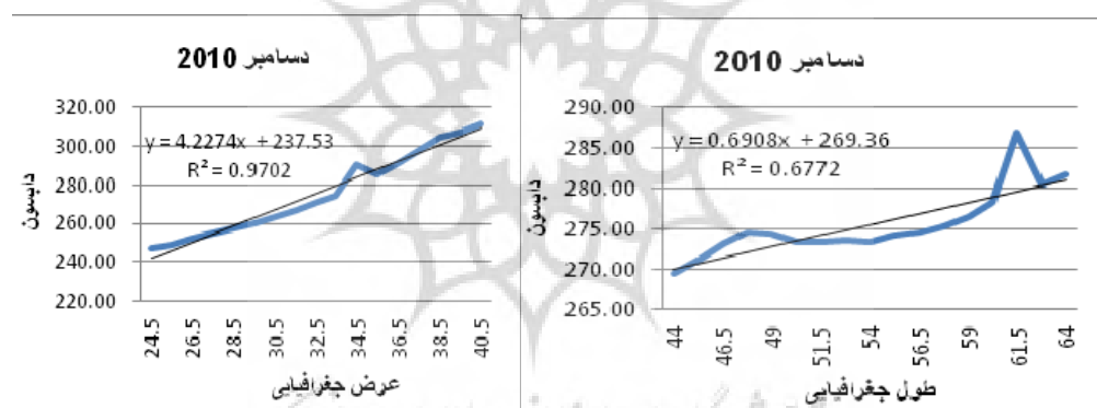
شکل ۶: روند تغییرات عرضی و طولی متوسط اُزون کلی در گستره‌ی ایران در دسامبر ۲۰۱۰
