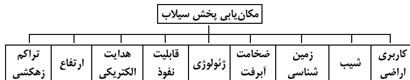
شکل (۴) نمایش دیاگرام پارامترها و معیارهای مورد مطالعه در مکان‌یابی پخش سیلاب
