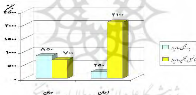
نمودار (۱) مقایسه پتانسیل بارندگی و تبخیر سالیانه ایران و جهان
