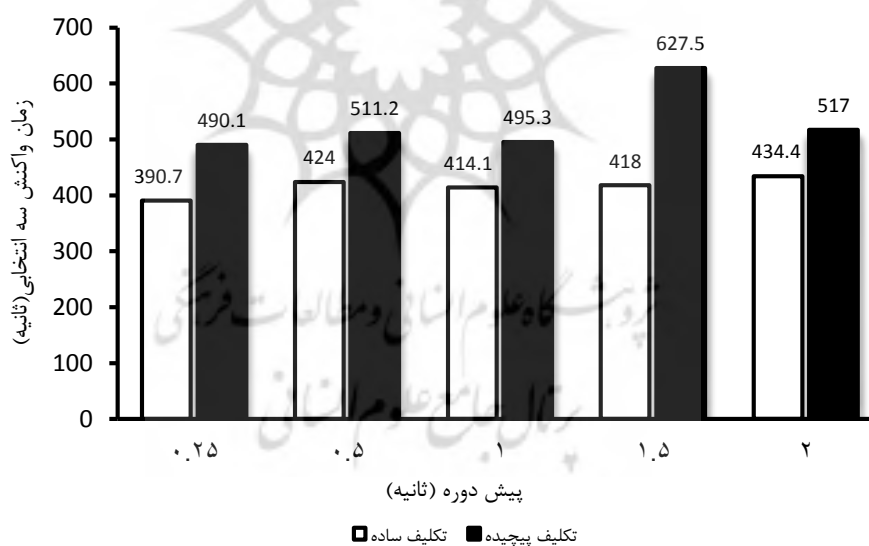
شکل ۳. نمودار زمان واکنش سه‌انتخابی تکلیف ساده و پیچیده
