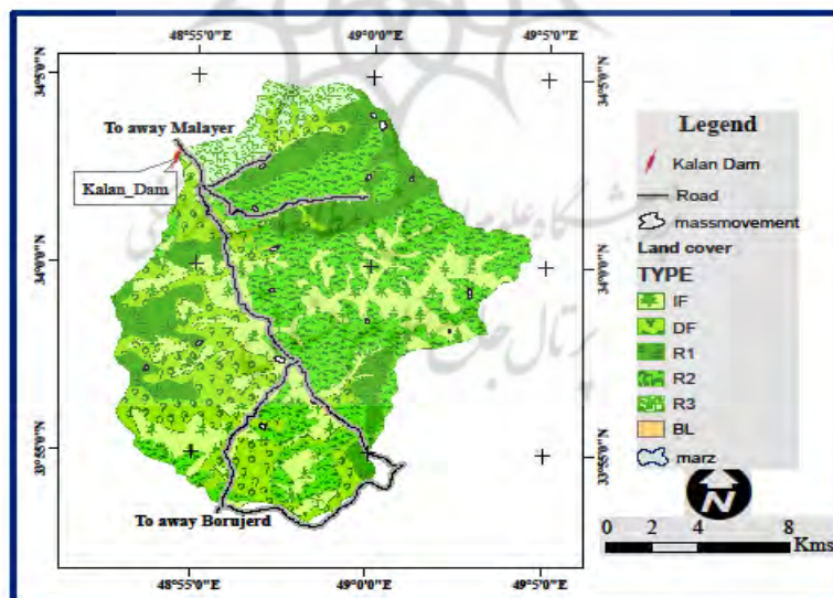
شکل (۸) نقشه تراکم پوشش گیاهی حوضه کلان مالیر
