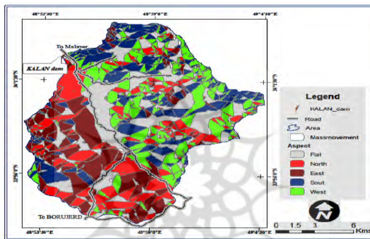
شکل (۶) نقشه جهت شیب حوزه کالان ملایر
