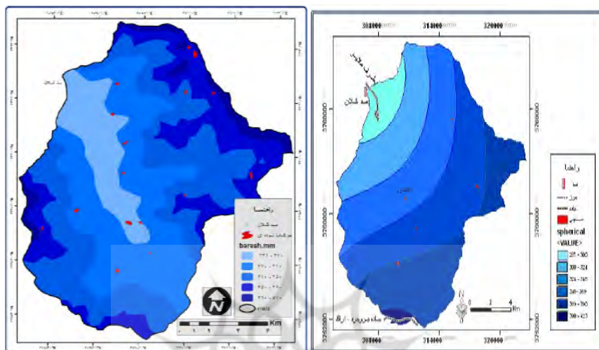
شکل الف (۱۰) نقشه طبقات همبران
