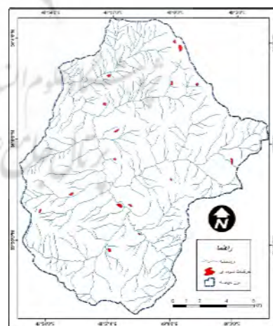
شکل (۲) الف- نقشه پراکنش حرکات توده‌ای
