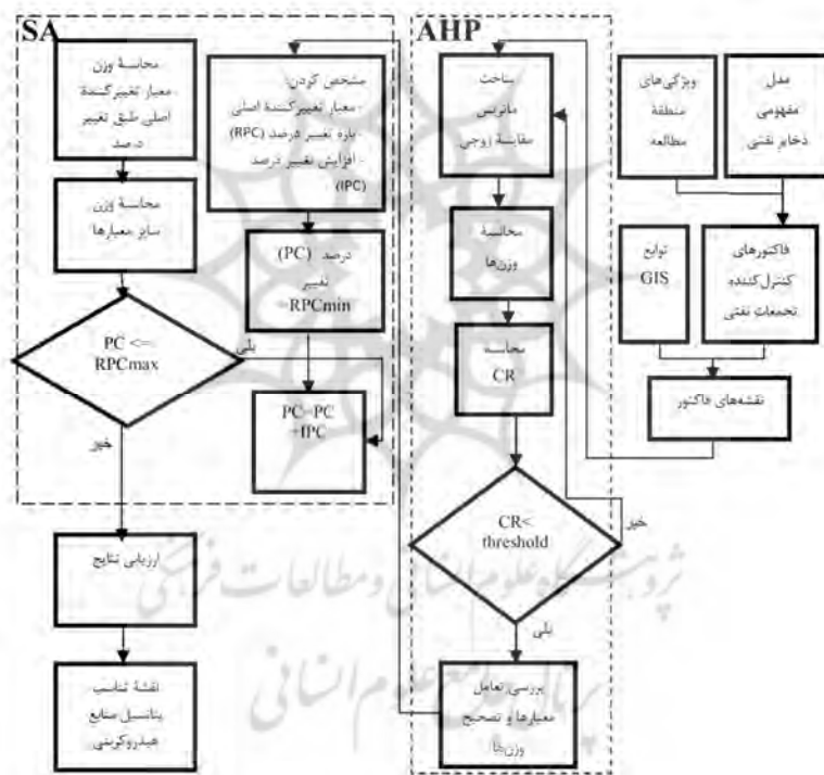
شکل 2 فلوچارت روش SA و AHP برای تهیه نقشه تناسب پتانسیل منابع هیدروکربنی
