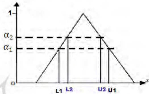
شکل ۲- بازه‌های ایجاد شده توسط \alpha_1 و \alpha_2
