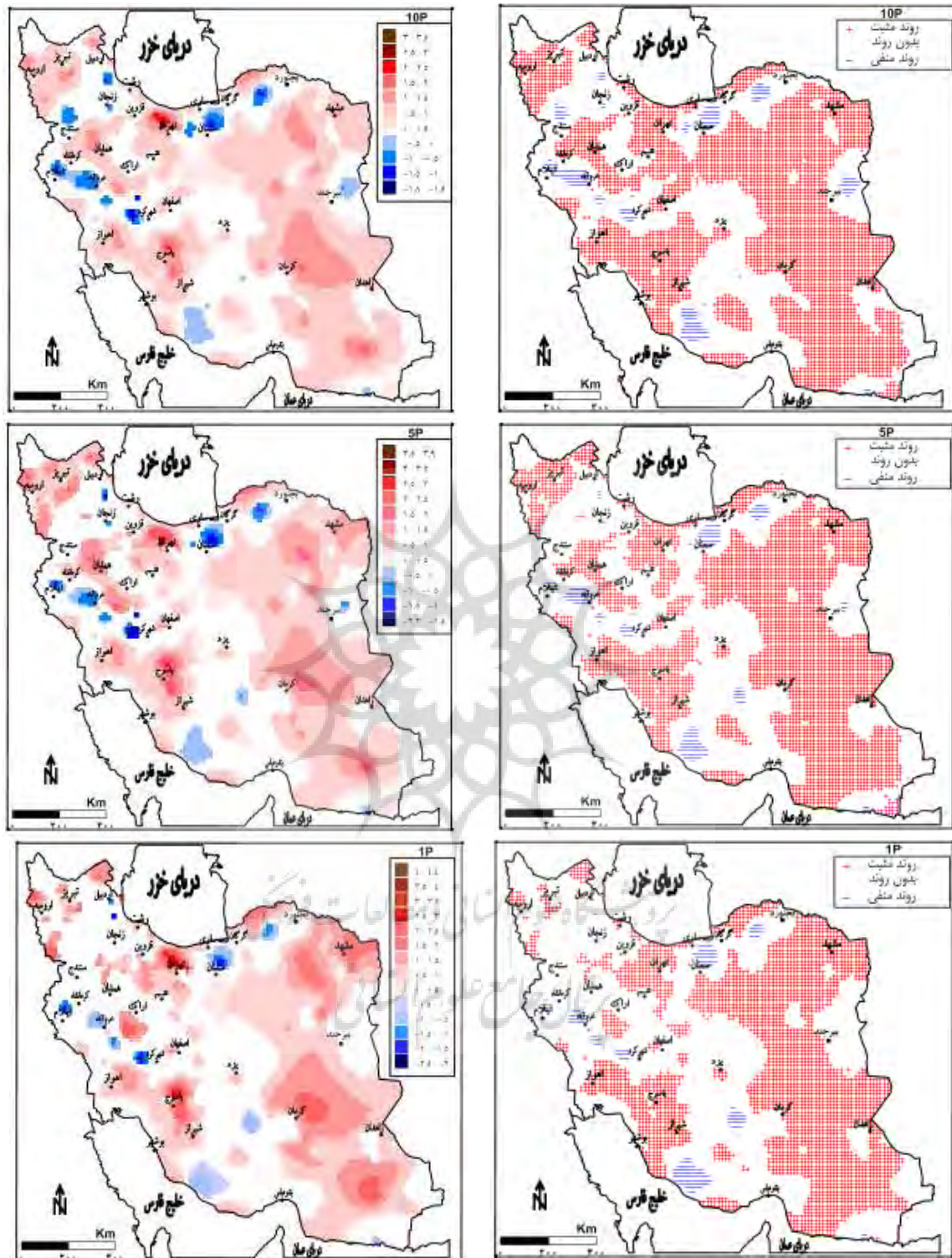
شکل ۱- روند نمایه‌های صدک ۱۰، ۵ و ۱م دمای کمینه (سمت راست) و مقادیر شیب روند (سمت چپ)
