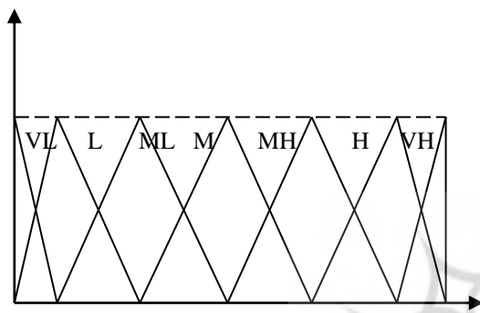
شکل شماره (۲): واژه های زبانی برای بیان اهمیت معیارها
