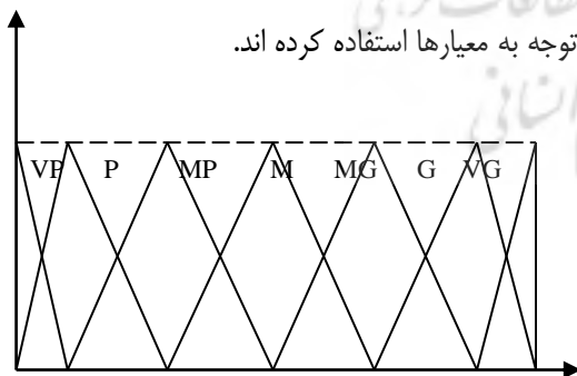
شکل شماره (۳): واژه های زبانی رتبه بندی گزینه ها
