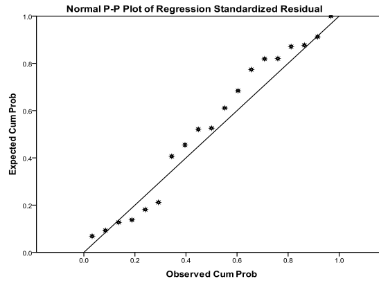
نگاره ۷: مدل رگرسیون P-P plot
