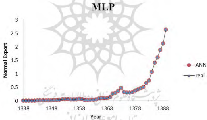
شکل (5): مقادیر واقعی و پیش‌بینی شده توسط مدل MLP برای دوره‌ی 1338-89 منبع: محاسبات تحقیق
