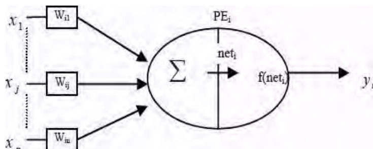
شکل (1): یک عنصر پردازشی
