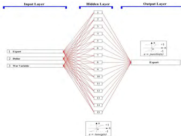
شکل (2): شبکه‌های پرسپترون چندلایه (MLP) مأخذ: نرم‌افزار مطلب
