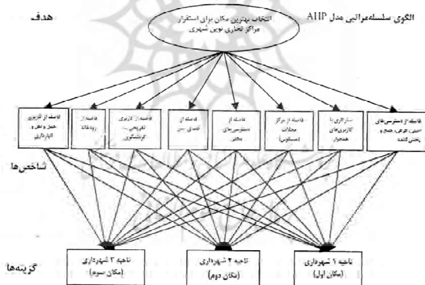
نمودار (۲) مدل تحلیلی AHP برای انتخاب بهترین مکان برای استقرار تجاری نوین شهری شهر سقز (ماخذ: نگارندگان)
