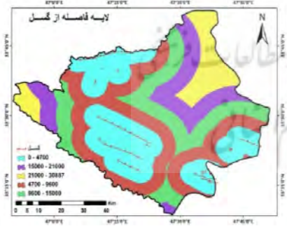
شکل (۸) لایه فاصله از گسل
