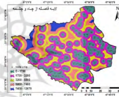
شکل (۵) لایه فاصله از چاه و چشمه
