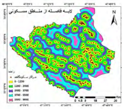
شکل (۳) لایه فاصله از مناطق مسکونی
