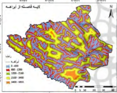
شکل (۶) لایه فاصله از آب‌راه
