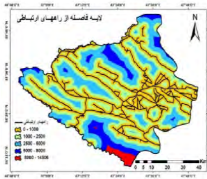
شکل (۴) لایه فاصله از راه‌های ارتباطی
