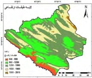
شکل (۹) لایه طبقات ارتفاعی منطقه
