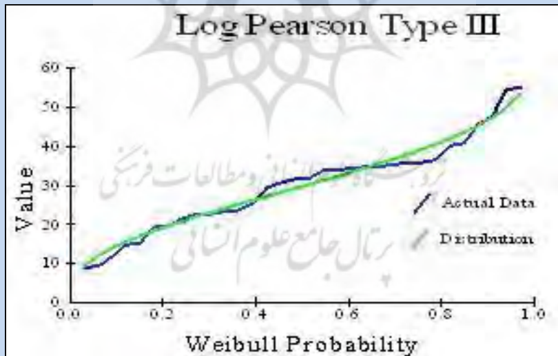
شکل شماره (7) برازش مدل توزیع احتمالی لوگ پیارسون تیسیم بر دادههای دبی حداکثر سالانه ایستگاه هیدرومتری تازهکند در سالهای آبی 1352-54
