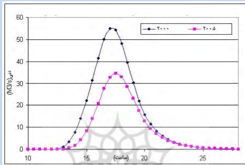
شکل شماره 8) نتایج شبیه‌سازی تأثیر تغییرات کاربری‌اراضی بر دبی پیک سیلاب براساس مقادیر CN سالهای 2000 و 2005 در ایستگاه تازهند صوفیجای
