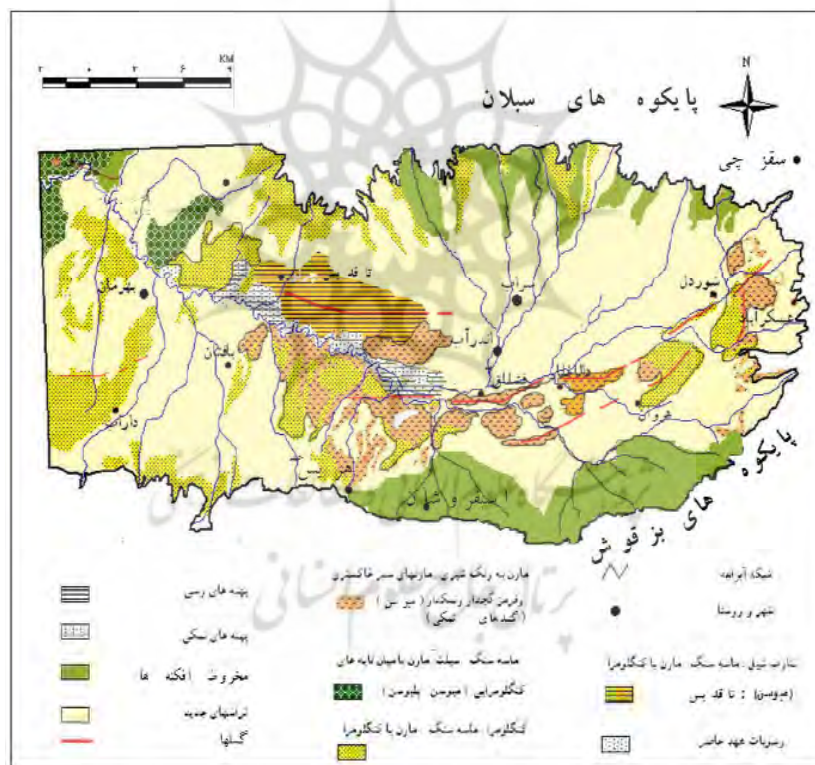
شکل (۴) نقشه زمین‌شناسی دشت سراب
