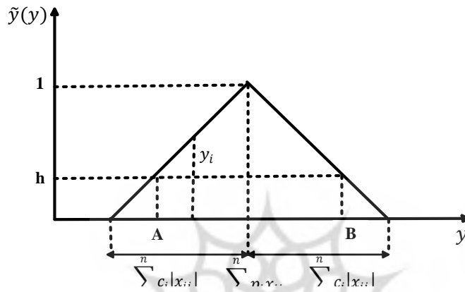
شکل ۲. تابع عضویت متغیر خروجی مدل رگرسیون
