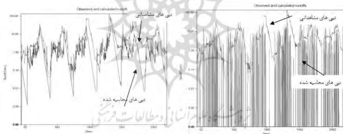
شکل (۳): نمودار رواناب مشاهداتی و محاسباتی برای حالت ۱۰۶
