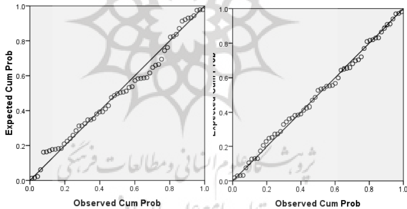
شکل ۲) پراکنش توزیع باقی مانده‌ها برای دمای خرم آباد
