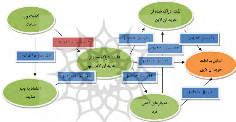
شکل ۲. مقادیر استاندارد مدل اولیه
