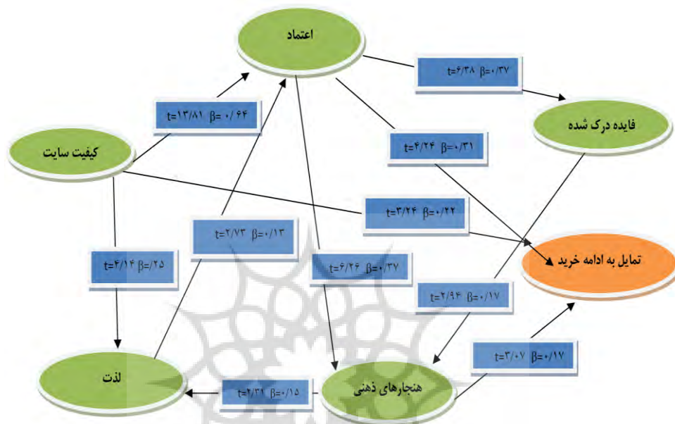
شکل ۳ مقادیر استاندارد مدل نهایی
