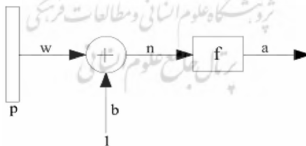
شکل (۲) مدل نرون تک ورودی
