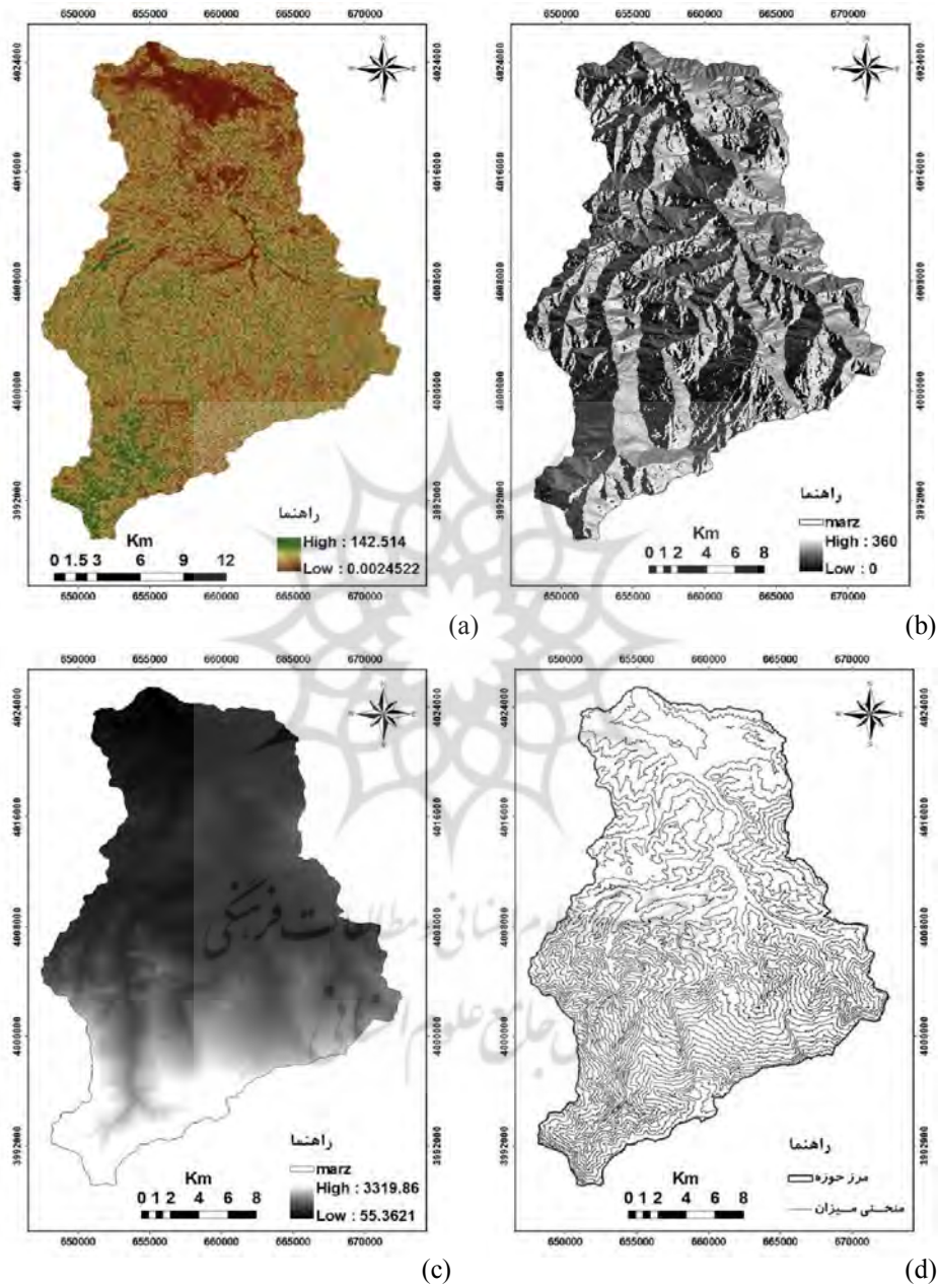
شکل (۲) اشکال مختلف منطقه مورد مطالعه: a: نقشه شیب، b: نقشه جهت، c: نقشه DEM و d: نقشه
