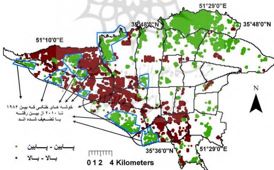
شکل (۸) پراکنندگی فضایی نقاط بالا-بالا و پایین-پایین برای دمای سطحی تهران در تاریخ ۱۹۸۶/۶/۲، قدرت تفکیک مکانی: ۱۲۰ متر
