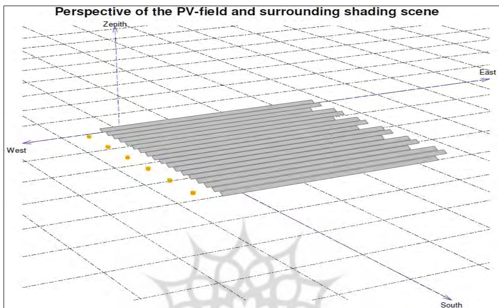
شکل ۱۳) نحوه چیدمان پانل‌ها در نیروگاه از دیدگاه سایه اندازی
