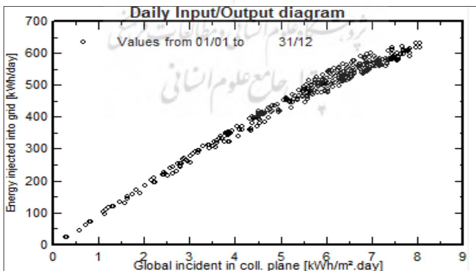
شکل ۹) نمودار پراکنندگی توزیع انرژی تزریق شده به شبکه به نسبت انرژی دریافت شده بر واحد سطح با شیب ۳۰ درجه
