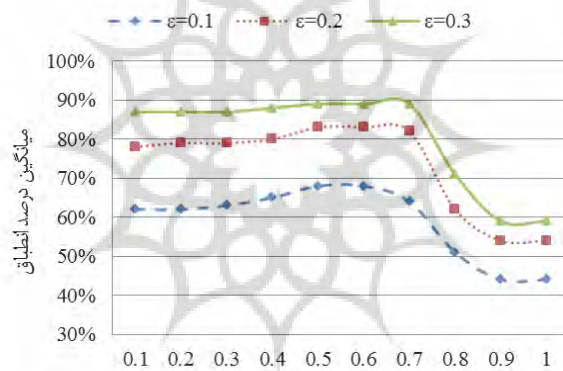
شکل ۱- نتایج حاصل از ارزیابی مدل با استفاده از روش شبیه‌سازی مونت کارلو
