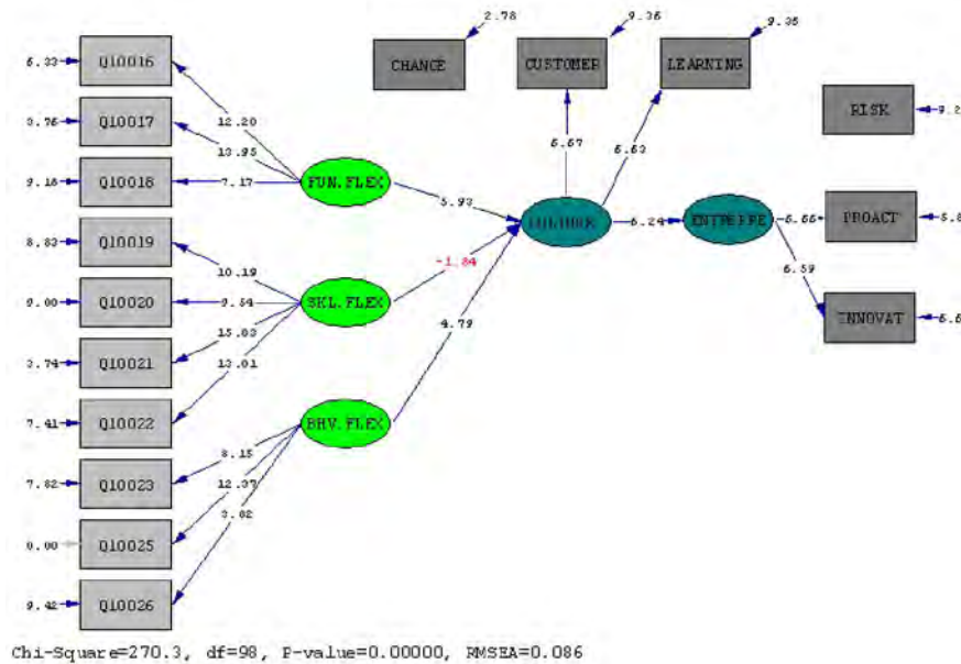
نمودار ۲: مدل‌سازی معادلات ساختاری (معناداری)
