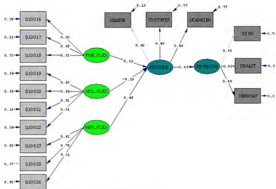
نمودار ۲: مدل‌سازی معادلات ساختاری (ضرایب استاندارد شده)
