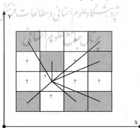
شکل ۴: نقشه شماتیکی از مدل‌سازی رستری با استفاده از روش درون‌یابی زمین‌آمار
