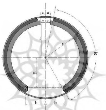
شکل ۳. طرح شماتیک سیستم ترمز کوپلینگ.
