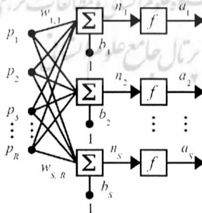
شکل ۶: شبکه‌ی عصبی تک‌لایه
