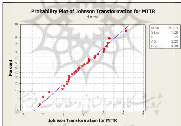
شکل ۵. نیکویی برآزش توزیع آماری نرمال برای داده‌های خط BMD2 تحت تبدیل جانسون
