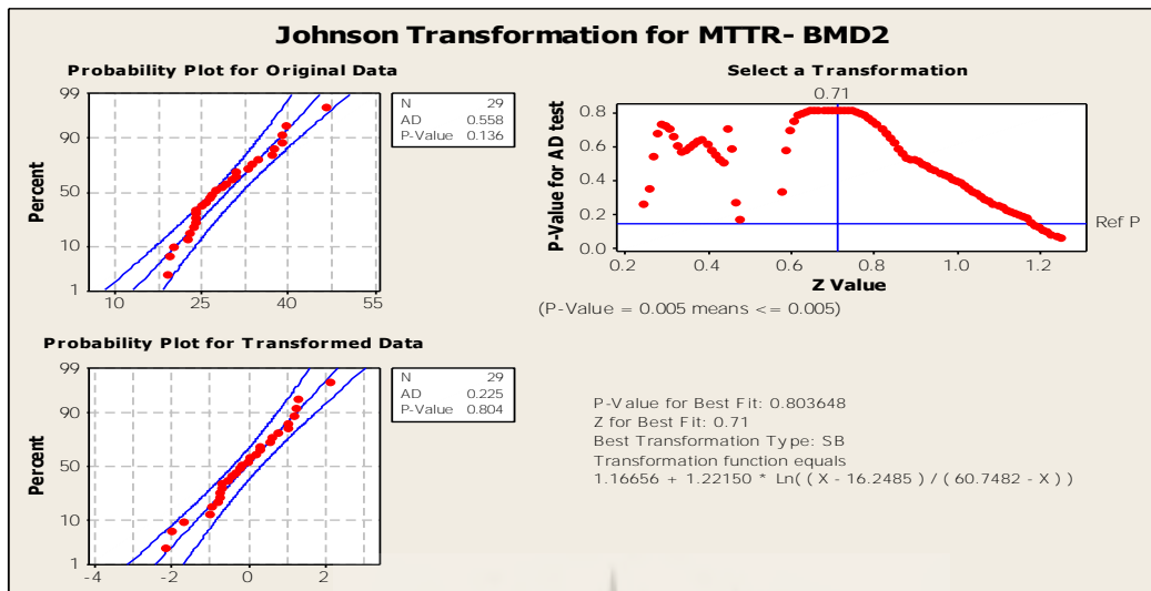
شکل ۴. نیکویی برآزش توزیع آماری نرمال برای داده‌های خط BMD2 تحت تبدیل جانسون
