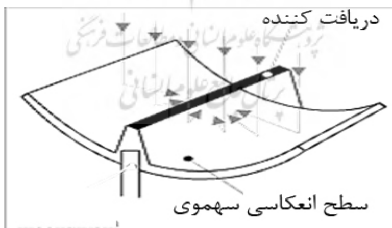
شکل ۶) طرح واژه کلکتور سهموی خطی خورشیدی [25]
