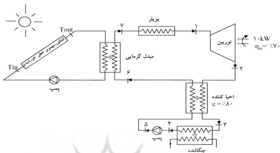
شکل ۵) طرح واژه چرخه رانکین آلی همراه با کلکتور سهموی خطی خورشیدی [14]
