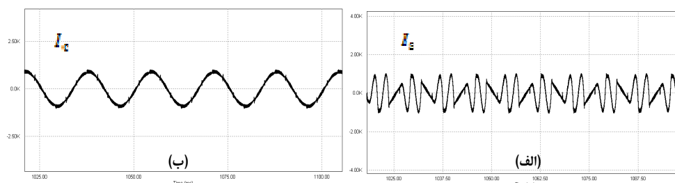
شکل ۱۳) روش ضریب توان واحد (UPF): (الف) جریان جبران سازی شده منبع، (ب) جریان تزریقی اینورتر
