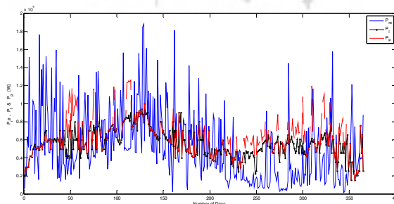
شکل ۲۱: توان تولیدی توسط سیستم ترکیبی خورشیدی-بادی-دیزلی ( P_p )، توان تولیدی توسط منابع تجدید پذیر ( P_{re} )، توان مورد
