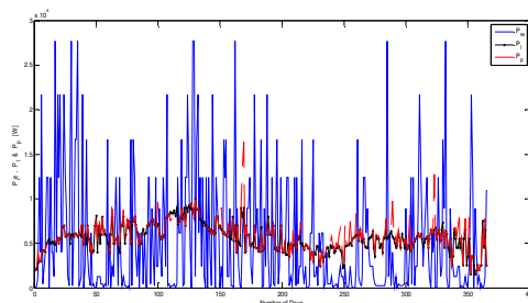
شکل ۱۶: توان تولیدی توسط سیستم ترکیبی بادی-دیزلی ( P_p )، توان تولیدی توسط منابع تجدید پذیر ( P_{re} )، توان مورد نیاز بار ( P_l )
