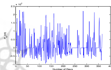
شکل ۱۷: توان ورودی / خروجی بانک باتری در طول سال
