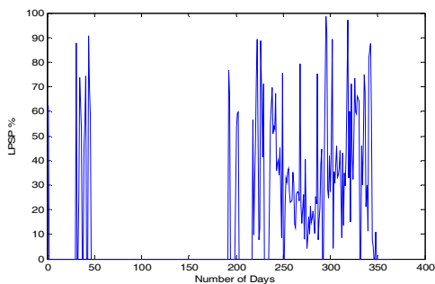
شکل ۱۵: شاخص قابلیت اطمینان سیستم ترکیبی خورشیدی-دیزلی
