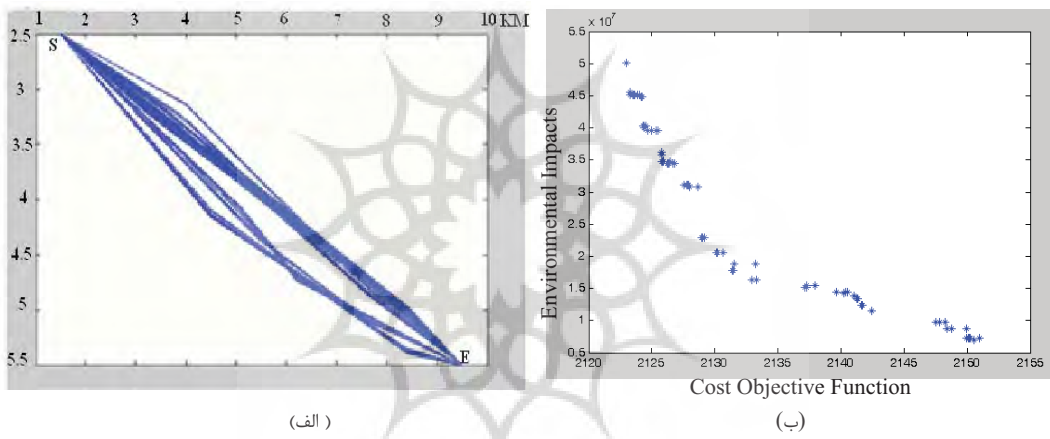
شکل ۴. نتایج اجرا با دو دکل کششی (الف) مسیرهای خطوط انتقال نیرو؛ (ب) مقادیر توابع هدف برای هر مسیر
