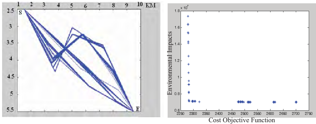
شکل ۶. نتایج اجرا با سه دکل کششی (الف) مسیره‌های خطوط انتقال نیرو؛ (ب) مقادیر توابع هدف برای هر مسیر (تعداد نسل ۲۰۰)
