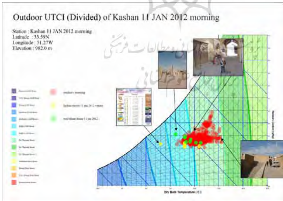
تصویر ۱۳: مقایسه وضعیت گرمایی گذرهای مختلف در صبح و ظهر زمستان با اقلیم محلی و شهری روی شاخص اقلیم دمایی جهانی
