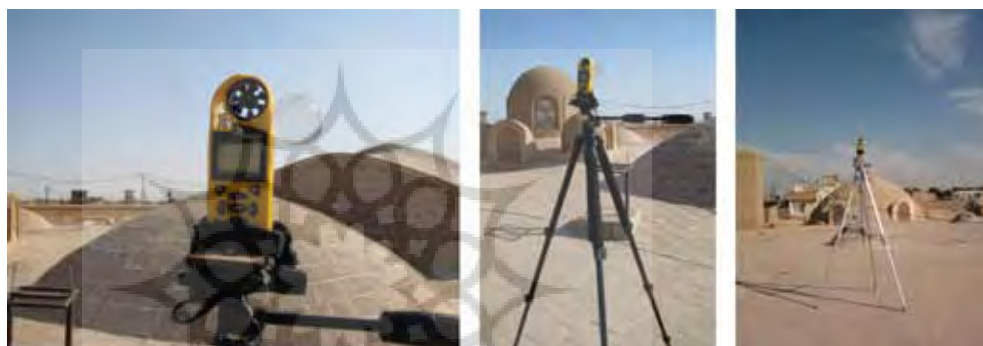
تصویر ۴: دستگاه هواشناسی مرجع روی بام خانه احسان (راست) و خانهٔ عامری‌ها (وسط و چپ)
