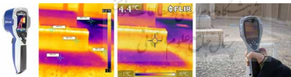
تصویر ۶: دوربین مادون قرمز FLIR i۷ و نمونه عکس‌های تهیه شده توسط آن
