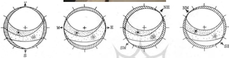
تصویر ۱۶: محدوده آسمان قابل رویت در گذرهای عریض و میدانچه‌ها روی نقشه مسیر خورشید
