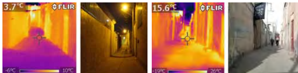
تصویر ۲۳: مقایسه وضعیت گرمایی گذر باریک شمالی / جنوبی در ظهر (راست) و شب (چپ) زمستان
