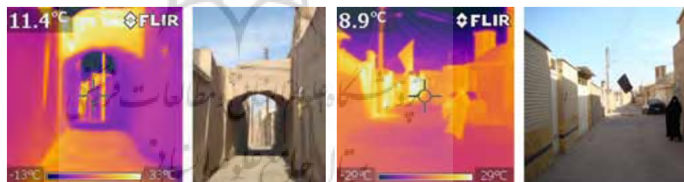
تصویر ۲۴: مقایسه وضعیت گرمایی گذرهای باریک سرباز (راست) و سرپوشیده (چپ) در زمستان
