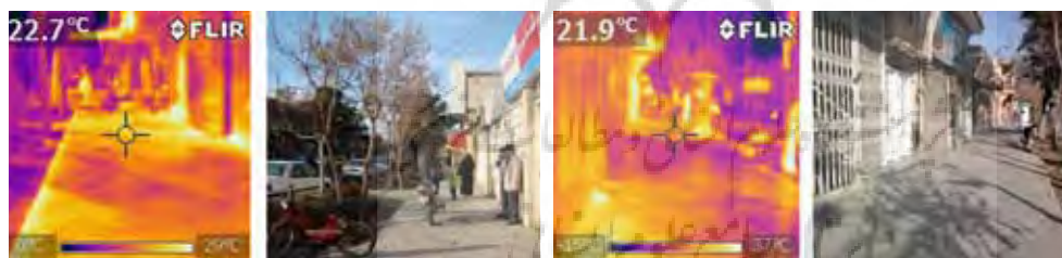
تصویر ۲۶: وضعیت گرمایی پیاده‌راه‌های خیابان‌های اصلی در ظهر زمستان
