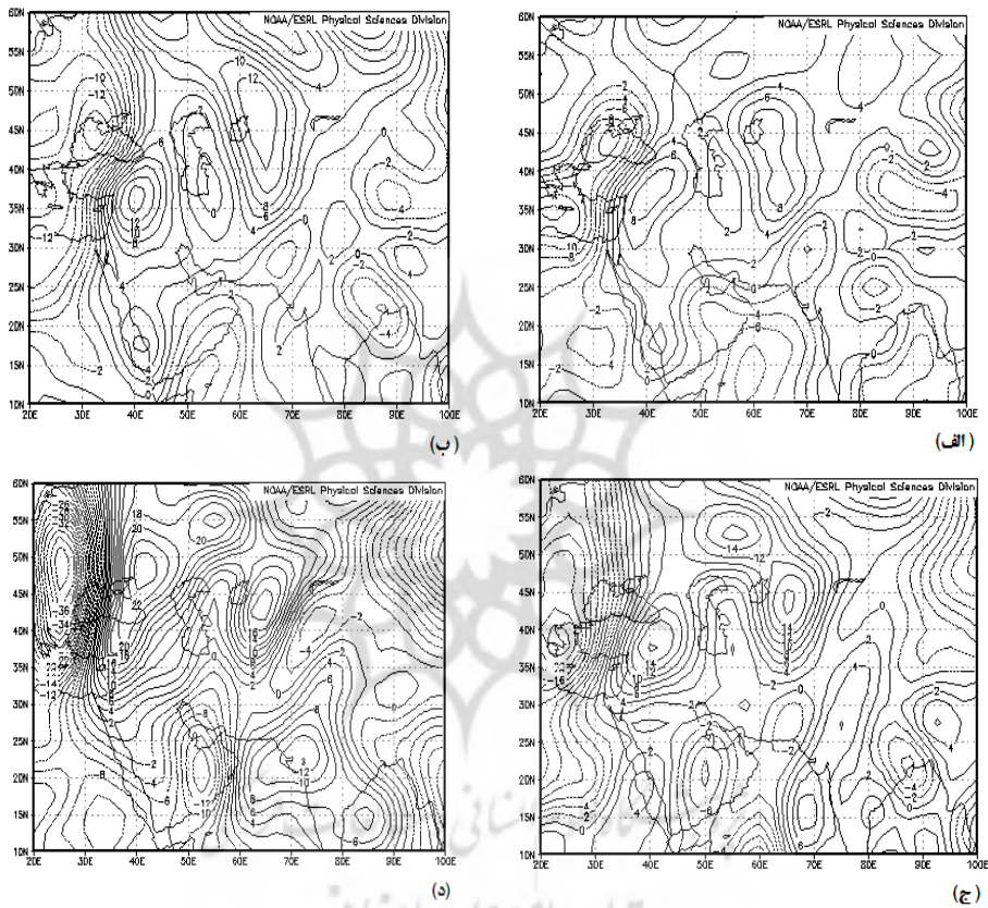
شکل ۸ نقشه مؤلفه نصف‌النهاری باد (V)، الف- سطح ۱۰۰۰، ب- سطح ۸۵۰، ج- سطح ۷۰۰، د- سطح ۵۰۰ هکتوپاسکال روز ۲۸ ژانویه ۲۰۰۷ ساعت ۱۲
