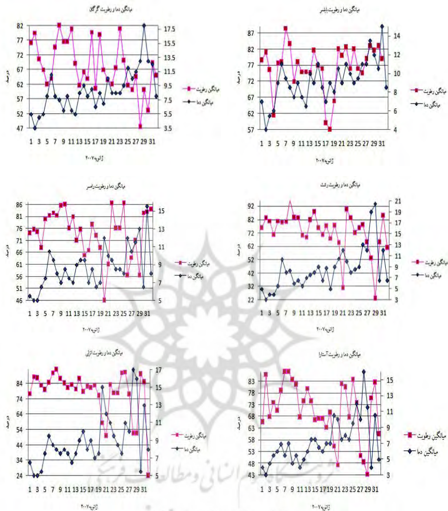
شکل ۳ مقایسه دما و رطوبت روزانه ایستگاه‌های سواحل خزر ژانویه ۲۰۰۷
